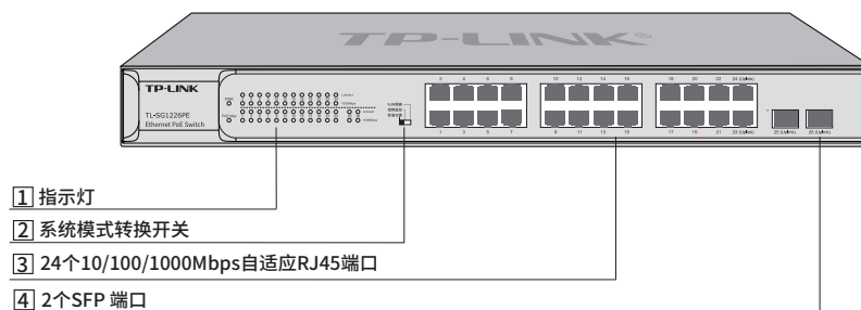
图1-3 TL-SG1226PE前面板示意图
